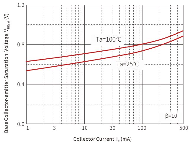
V_{BE\text{sat}} \text{ — } I_C
