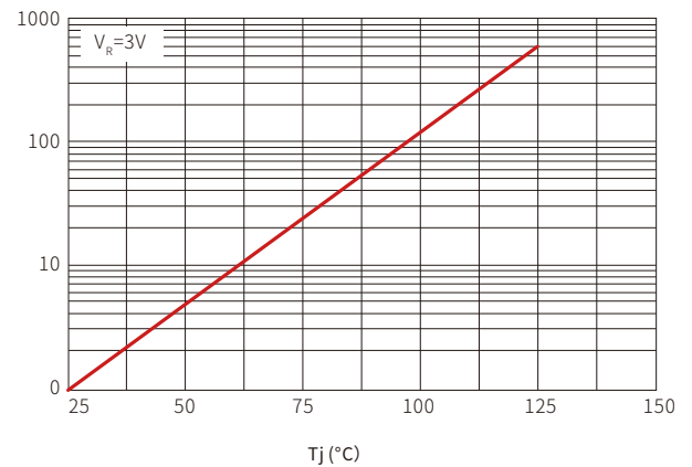
Fig.4 I_R(T_J)/I_R(T_J=25^\circ\text{C})
