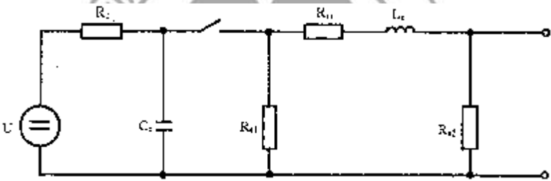
U—高压源;R c —充电电阻;C c —储能电容;R s —脉冲持续时间形成电阻; R m —阻抗匹配电阻;L r —上升时间形成电感
