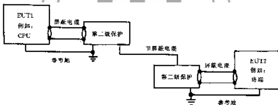
图 B2 在公共参考地系统分开的大楼内实现第二级浪涌保护的示例
